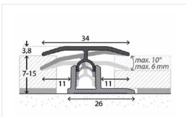
34 mm leveät alakiskolistat metallipinnalla. 7–15 mm pintamateriaaleille.
