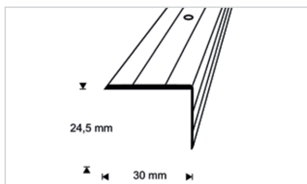
Askelkulmat 30 x 24,5 mm, ruuvikiinnitys (voi kiinnittää myös porrastasanteille etureunasta ruuvattuna)
